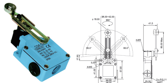
CSA-031
