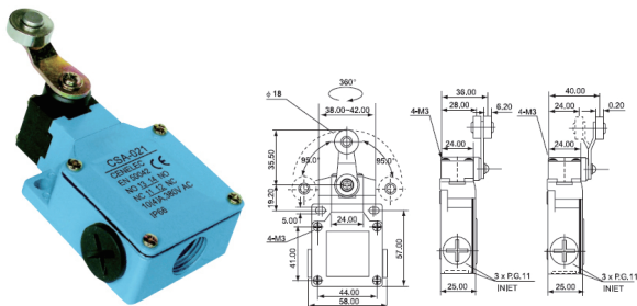
CSA-021
