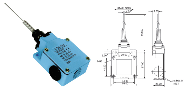
CSA-061
