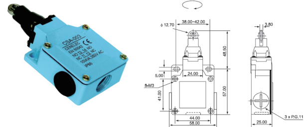
CSA-003
