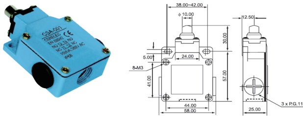
CSA-001
