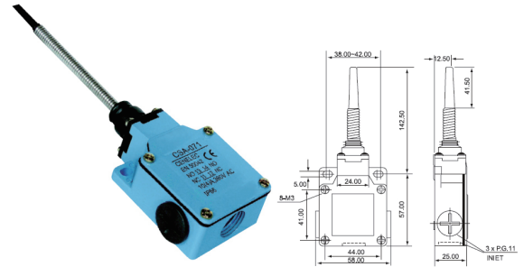
CSA-071
